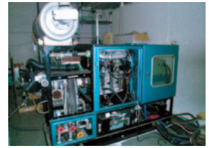
バイオガス専燃コージェネレーションシステムの開発 (ロータリーエンジン)
